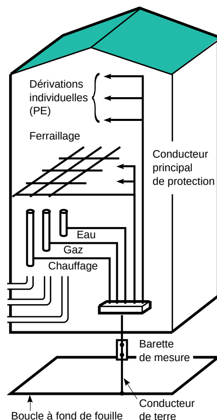
Fig. 4 : équipotentialité dans un immeuble.
