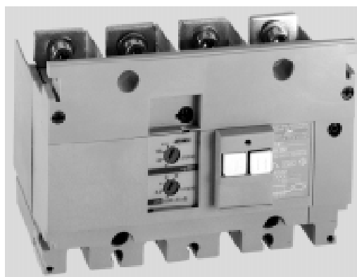
Fig. 23 : bloc vigi de Compact NS.
