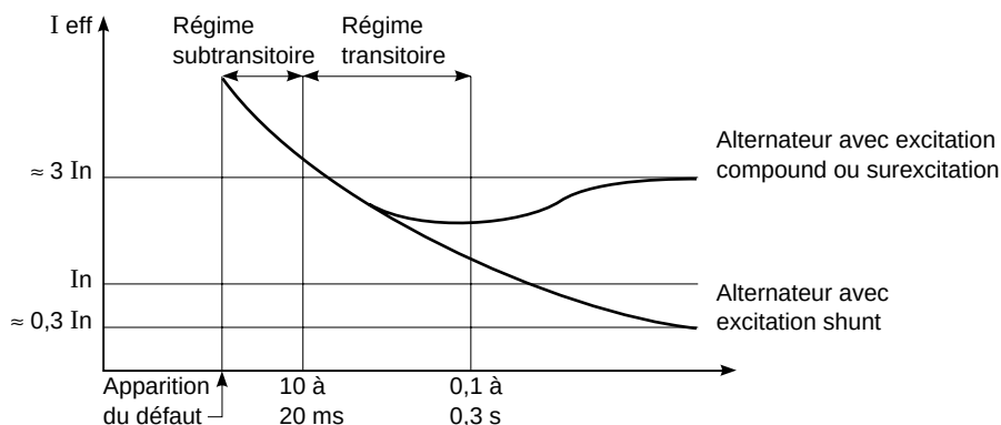
Fig. 17 : établissement d'un courant de court-circuit dans un réseau alimenté par un groupe de secours « diesel/alternateur ».
