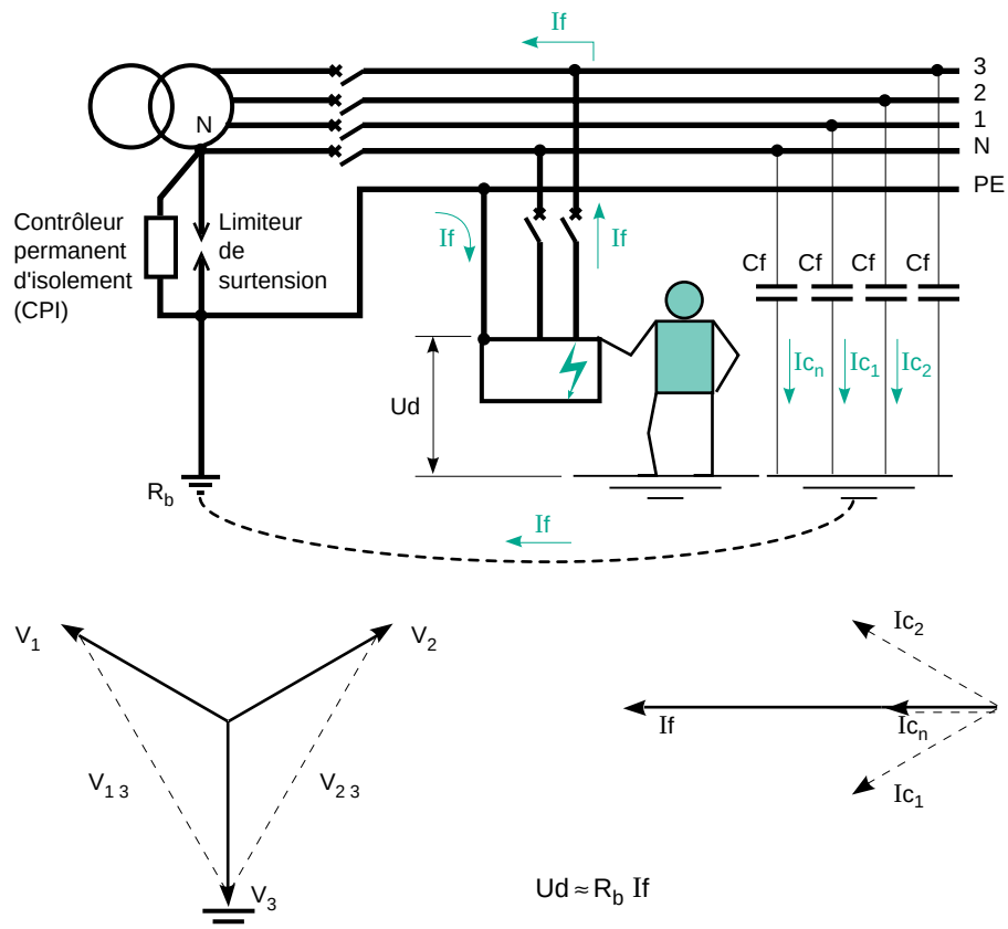
Fig. 12 : courant de premier défaut d'isolement en schéma IT.
