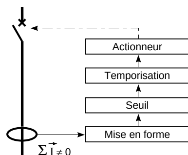
Fig. 24 : schéma fonctionnel d'un DDR.
