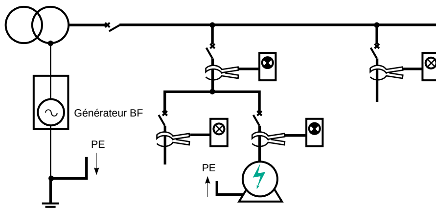
Fig. 26 : localisation du défaut d'isolement par suivi du trajet d'un courant basse fréquence injecté à l'origine de l'installation.
