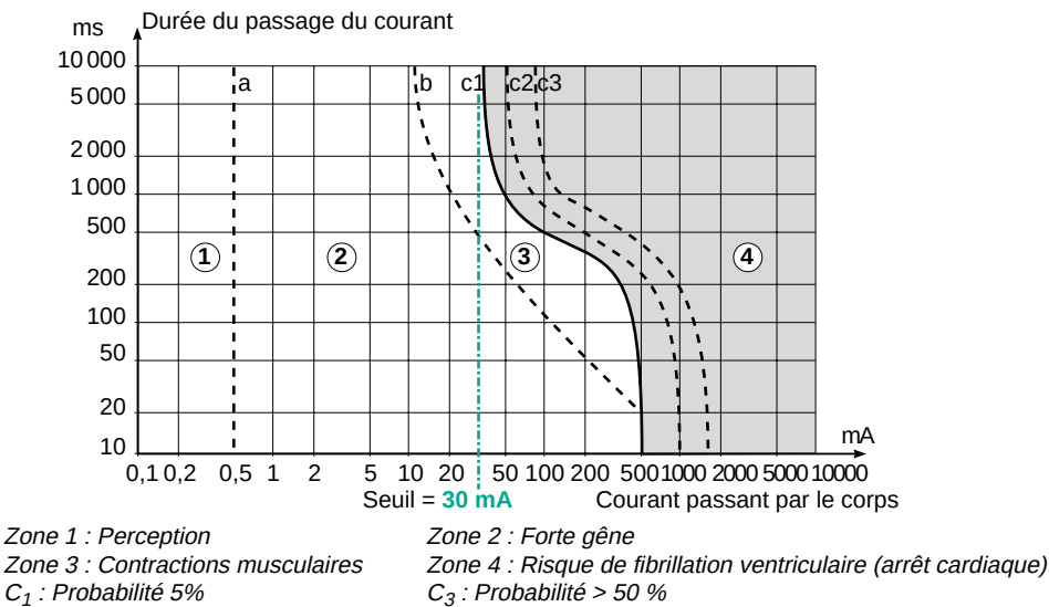
Fig. 1 : zones temps/courant des effets du courant alternatif (15 Hz à 100 Hz) sur les personnes selon la norme CEI 60479-1.
