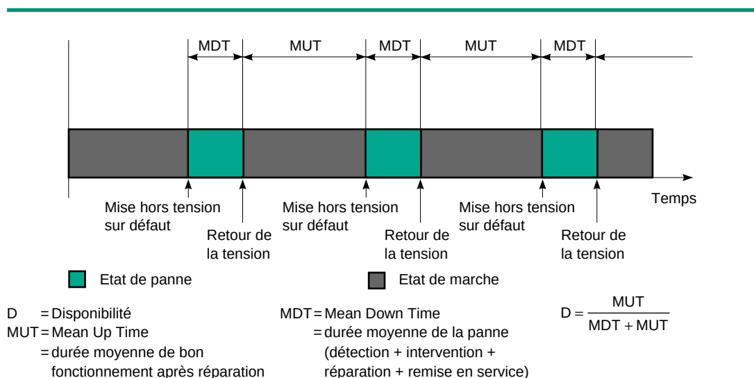
Fig. 16 : disponibilité de l'énergie électrique.
