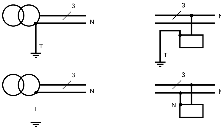
Fig. 5 : mode de raccordement, à la terre du neutre du transformateur, et des masses des récepteurs électriques.
