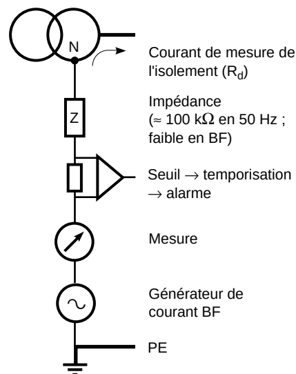
Fig. 25 : schéma fonctionnel d'un contrôleur permanent d'isolement (CPI).
