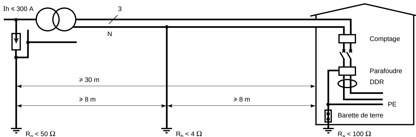
Fig. 20 : distribution publique aérienne rurale en France.
