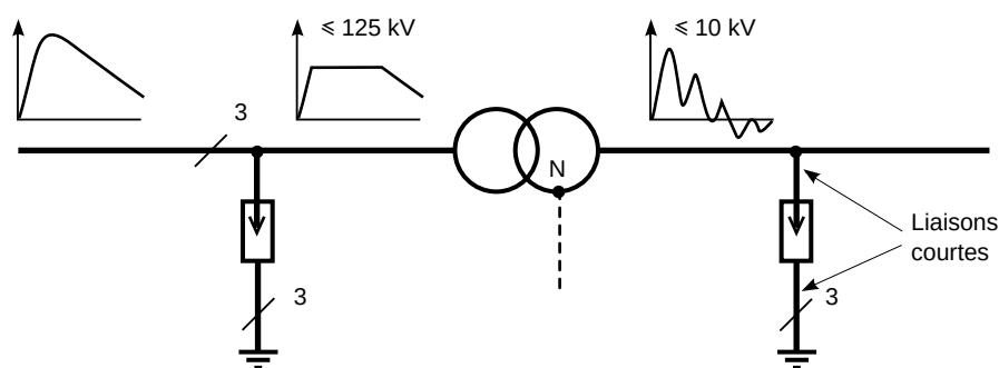
Fig. 18 : limitation et transmission des surtensions de foudre (que le neutre soit à la terre ou non, il y a des surtensions de mode commun sur les phases).
