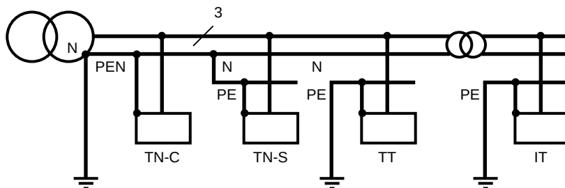
Fig. 6 : exemple de coexistence entre les divers SLT.
