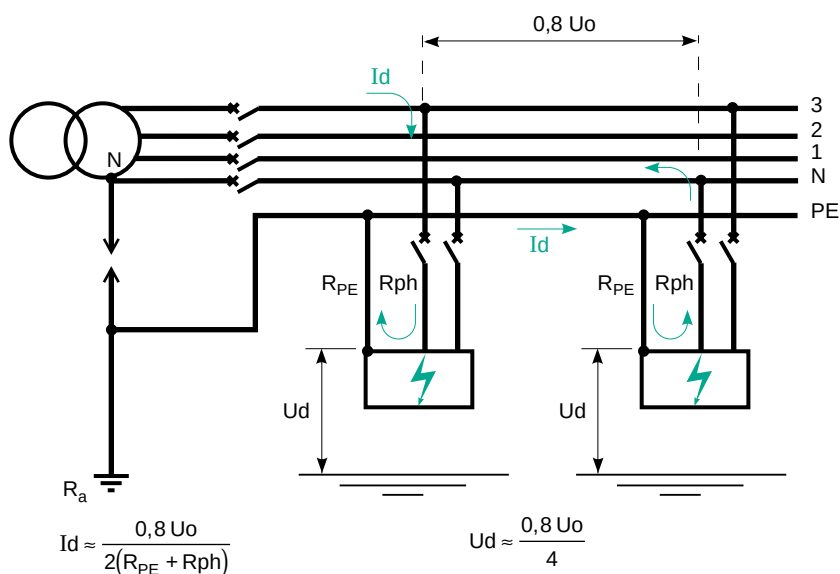
Fig. 13 : courant de 2 ème défaut en schéma IT (neutre distribué) et départs concernés de même section et même longueur.
