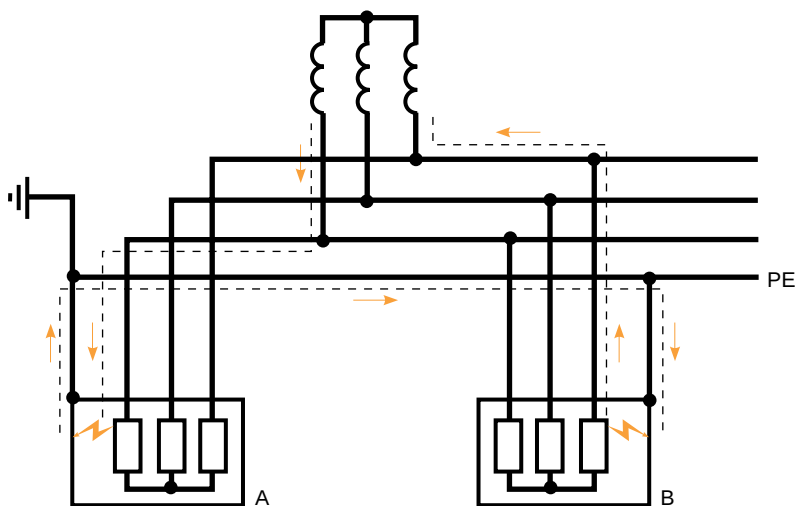
fig. 8 : schéma IT.
