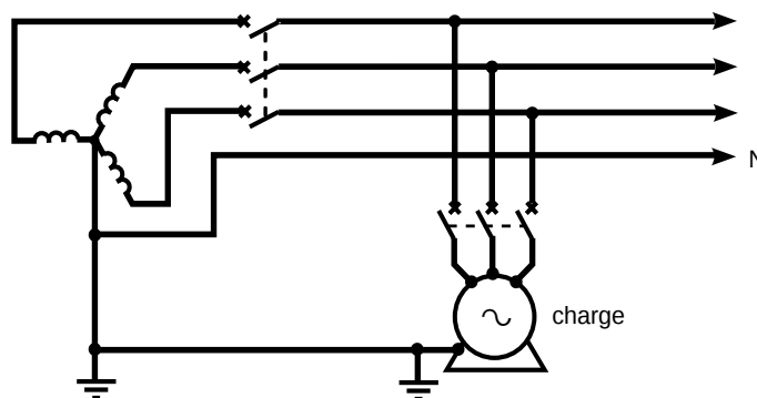
fig. 13 : schéma du SLT TN-S aux USA.
