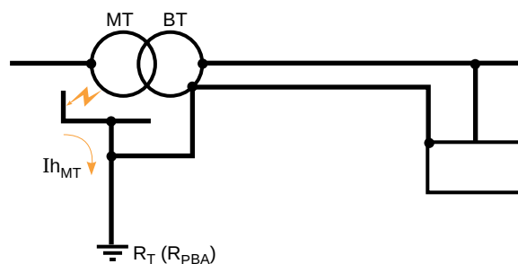
fig. 9b : les masses des récepteurs BT sont portées au potentiel I_{h_{MT}} \cdot R_T .
