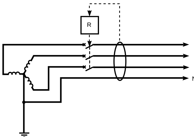
fig. 16 : zéro séquence.
