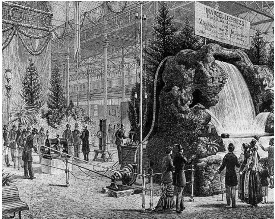
fig. 1 : installation de M. Desprez dans le palais de l'exposition de Munich.
