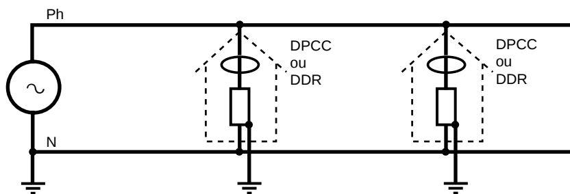
fig. 4 : neutre à la terre en distribution publique monophasée.
