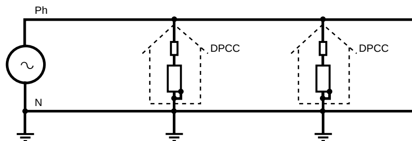
fig. 5 : neutre TN-C en distribution publique monophasée.
