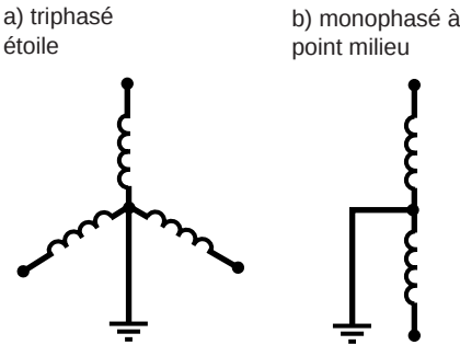
fig. 11 : couplage des enroulements secondaires du transformateur MT/BT.
