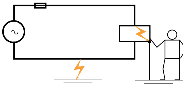
fig. 2 : à l'origine : l'émergence du neutre isolé.
