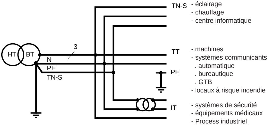
fig. 24 : coexistence de plusieurs SLT dans une installation BT.
