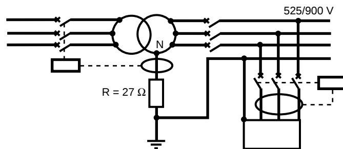
fig. 18 : SLT utilisé en RSA.
