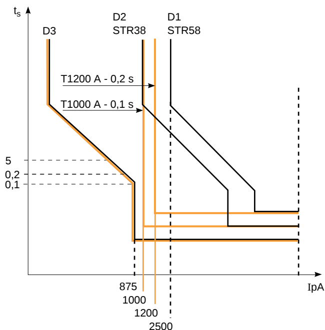
fig. 17 : sélectivité entre protection contre les courts-circuits aval (D3) et protections de terre (GFP) amont, en orange.
