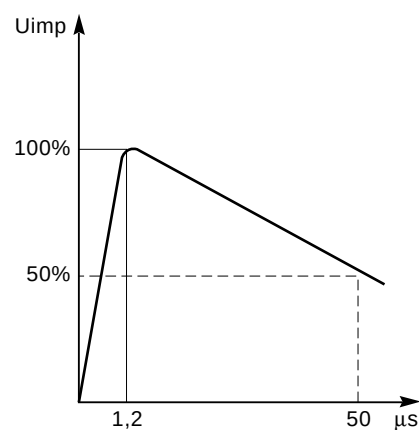
fig. 10 : onde de choc pour les disjoncteurs industriels 1,2 / 50 \mu s .
