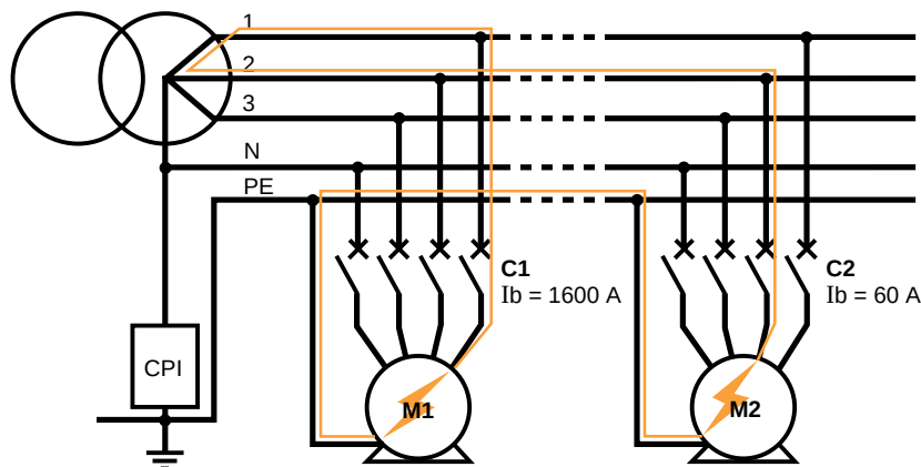
fig. 5 : exemple de coupure d'un courant de «double défaut» dans une installation en schéma IT. Du fait de la différence de calibres entre deux disjoncteurs (C1 et C2), il est possible qu'un seul (C2) soit en position d'éliminer le défaut avec un seul pôle sous la tension composée (phase/phase).
