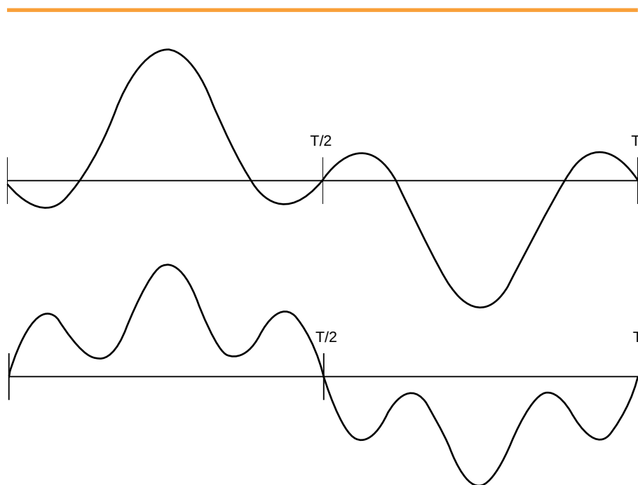
fig. 14 : formes d'ondes appliquées aux appareils pour les tests d'immunité aux harmoniques.
