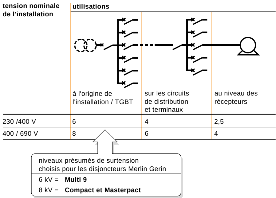
fig. 11 : niveaux présumés de surtensions transitoires (suivant publication 38 de la CEI et NF C 15-100 édition 1990, pour une altitude de 2000 m).
