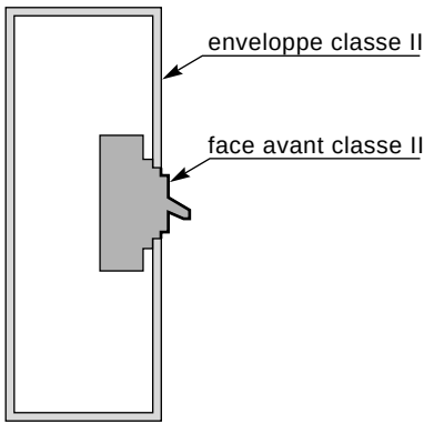
fig. 13 : équipement de classe II avec disjoncteur de classe II en face avant.
