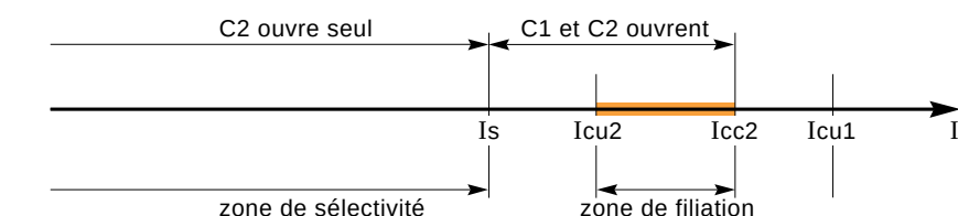
fig. 7 : principe de filiation entre deux disjoncteurs, l'appareil C2 dont le pouvoir de coupure I_{cu2} est inférieur au courant de court-circuit triphasé à ses bornes ( I_{cc2} ), est protégé ou «aidé» par l'appareil C1.
