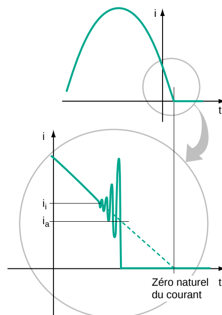
Fig. 9 : schéma d'un circuit lors de la coupure d'un faible courant inductif.
