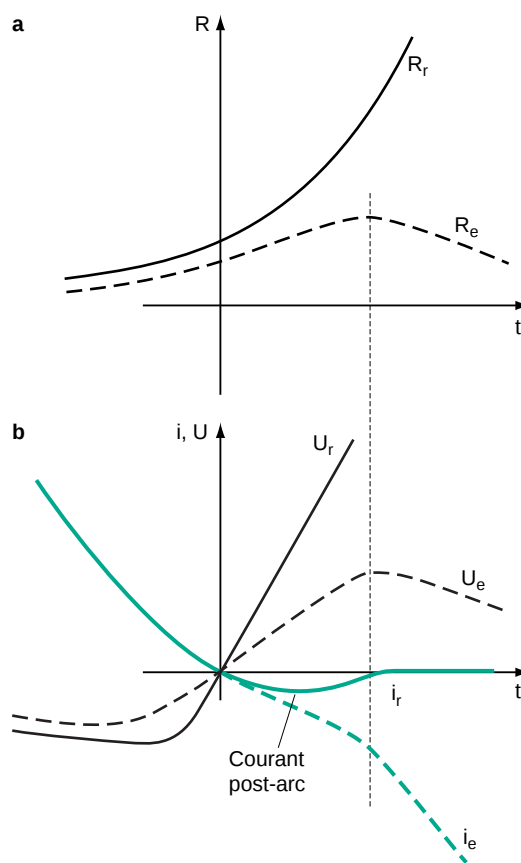
Fig. 5 : évolution de la résistance d'arc [a] et de la tension et du courant [b] pendant la période d'extinction, en cas de coupure réussie (r) ou d'échec thermique (e).
