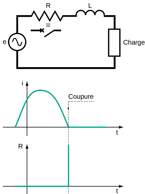
Fig. 3 : coupure réalisée par un interrupteur idéal.
