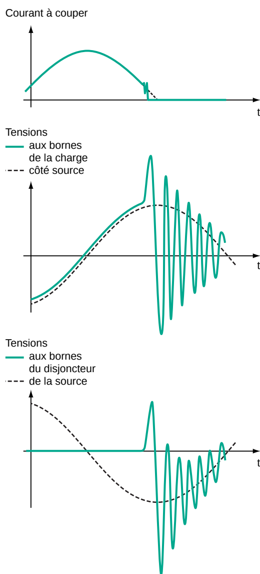
Fig. 11 : courbes de courant et de tension lors de la coupure de faibles courants inductifs.
