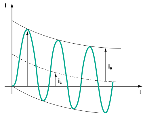
Fig. 16 : lors d'un court-circuit, le courant est la somme de deux composantes, l'une symétrique ou périodique ( i_a ) et l'autre asymétrique ou apériodique ( i_c ).
