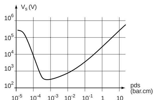
Fig. 20 : évolution de la rigidité diélectrique de l'air en fonction de la pression, en champ faiblement hétérogène (courbes de Paschen).
