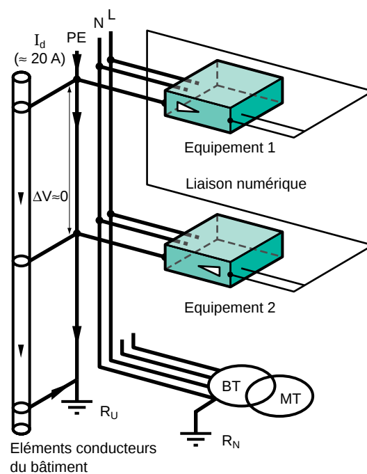
fig. 24 : schéma TT ; le faible courant dans le PE ne perturbe pas l'équipotentialité des références de potentiel des électroniques communicantes ( R_{PE} faible devant R_U et R_N , et I_d faible) les champs magnétiques et les \Delta V sont 1000 fois plus faibles qu'en TN-C ou TN-S.
