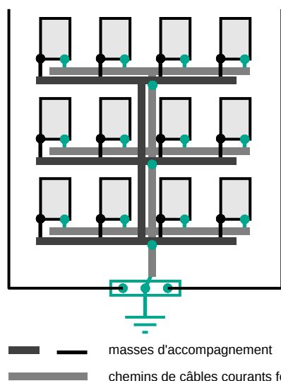
fig. 27 : recherche de l'équipotentialité en BF et HF.
