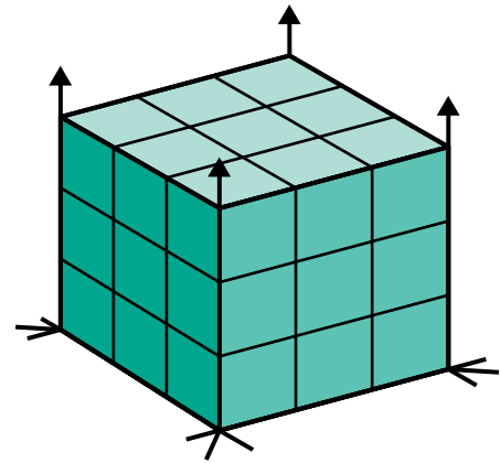
fig. 14 : maillage horizontal et vertical du bâtiment. Il constitue une cage de Faraday.
