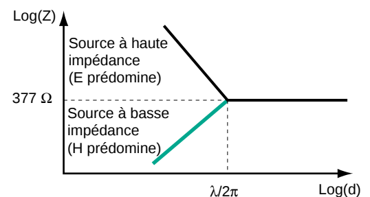
fig. 1 : impédance d'onde Z = f(d) .
