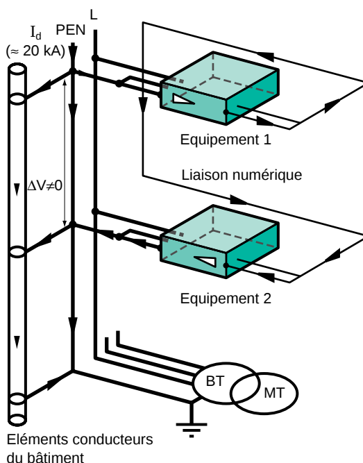
fig. 22 : schéma TN-C avec maillage ; le \Delta V permanent (déséquilibre, harmoniques multiples de 3) et temporaire (défaut) est atténué ; mais « courants vagabonds » : risque d'incendie et champs magnétiques perturbateurs, y compris au niveau des câbles de puissance (cf. fig. 20 ).
