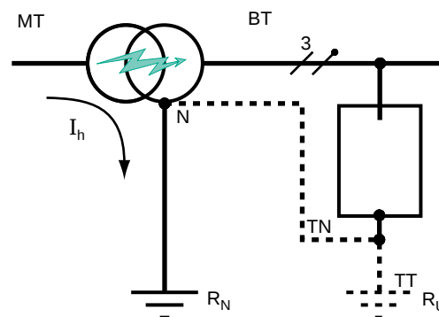
fig. 8 : claquage MT/BT ; le réseau monte en potentiel par rapport à la terre ; U = R_N \cdot I_h d'où risque pour le matériel en schéma TT ou pour les personnes en schéma TN si le bâtiment n'est pas totalement équipotentiel.
